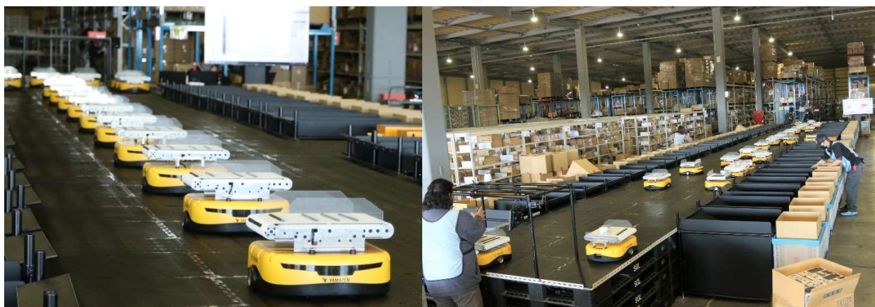
t-Sort cb15と周辺機材を工夫し組み合わせ、山善と+A 共同で様々な日用品の仕分け自動化を実現
